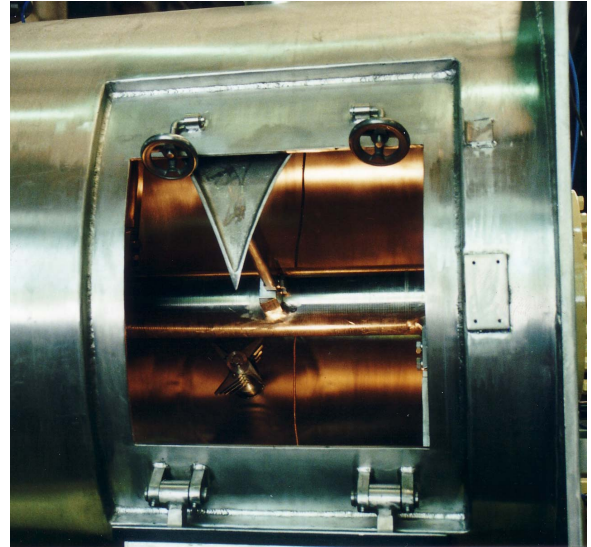
Detalle de pala de arado y disgregador en mezcladora de acero inoxidable con camisa de calefacción
