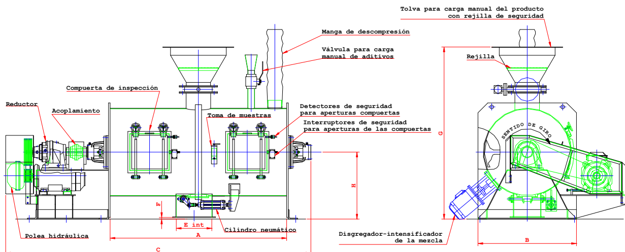
Mezcladora MT-200 de 2.000 l de capacidad construida en acero al carbono
