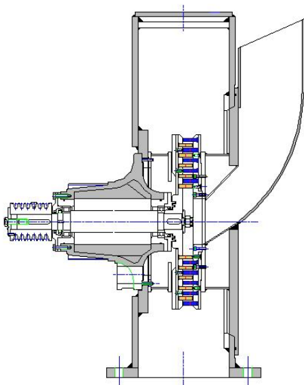
Corte seccional molino DÚPLEX tipo AP, equipado con pitones
