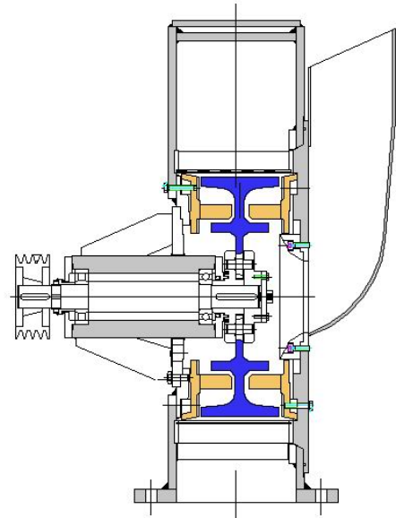
Corte seccional molino DÚPLEX tipo AM, equipado con martillos
