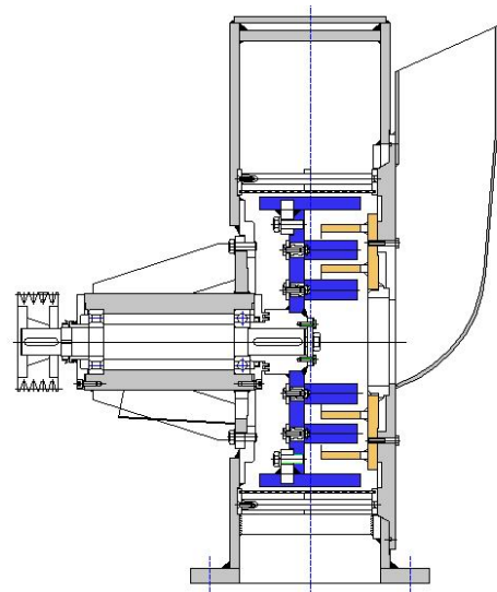
Corte seccional molino DÚPLEX tipo AME, equipado con batidores
