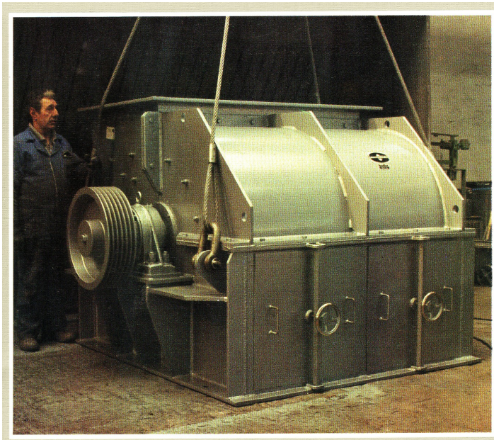
Molino de martillos, modelo MM-10
